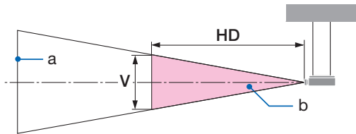
a: Leinwand / b: Gefahrenbereich
