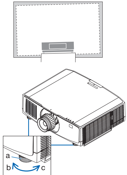
a: Neigungsfuß/b: Nach oben/c: Nach unten
