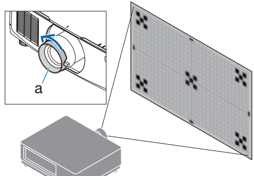
a: Verzerrungsring
