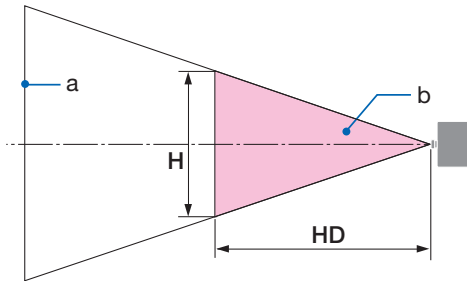
a: Leinwand / b: Gefahrenbereich
